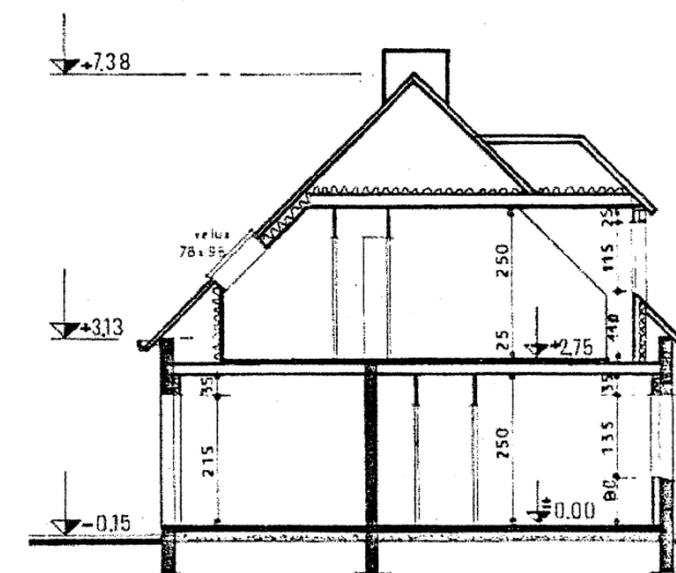
— COUPE SCHÉMATIQUE AA —
