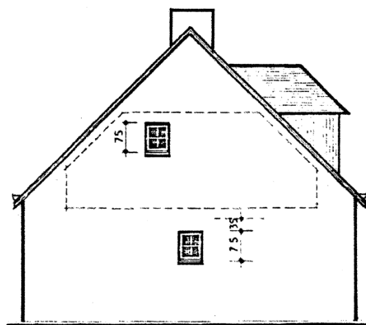
PIGNON GAUCHE
