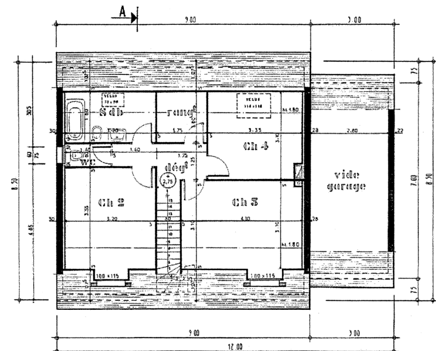
PLAN DE L'ÉTAGE
